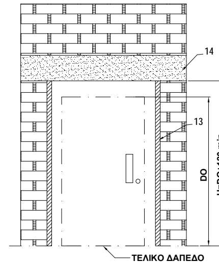
ΤΥΠΙΚΗ ΔΟΜΗΣΗ ΕΙΣΟΔΟΥ ΑΝΕΛΚΥΣΤΗΡΑ ΜΕ ΠΛΙΝΘΟΔΟΜΗ
